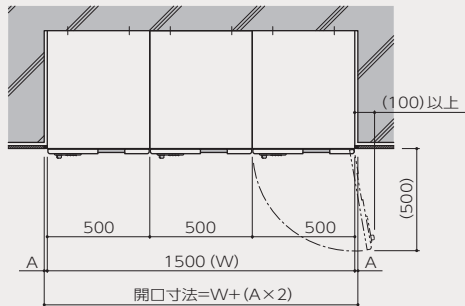
平面
