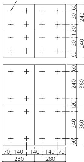
●アンカーピッチ図
