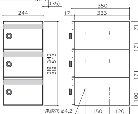
●施工図
