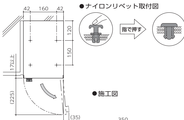
●ナイロンリベット取付図
