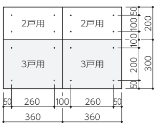
○ヨコ型 (F1053Y-2・3)
