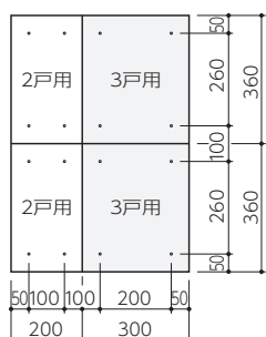
○タテ型 (F1053T-2・3)
