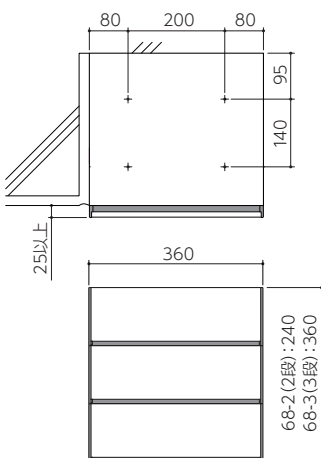
●施工図
