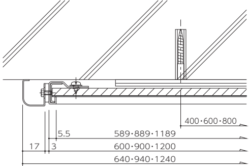
平断面
