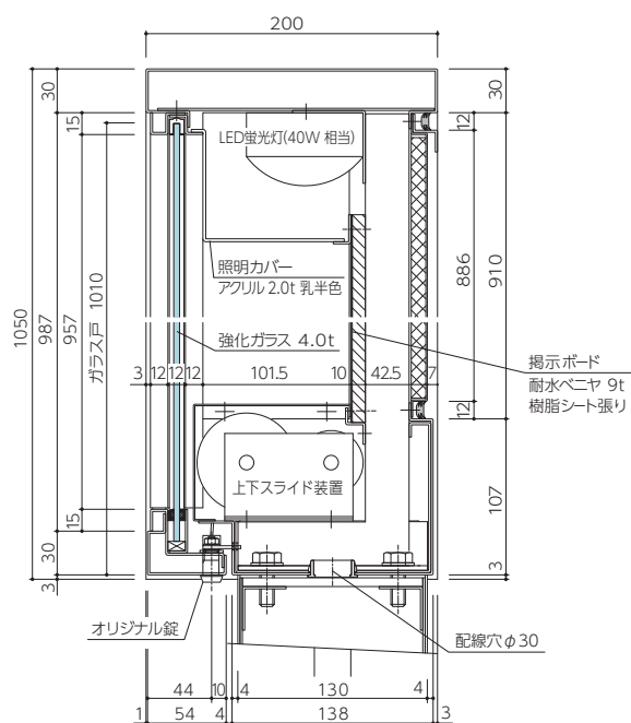
立断面
