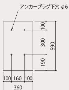
アンカーピッチ図
