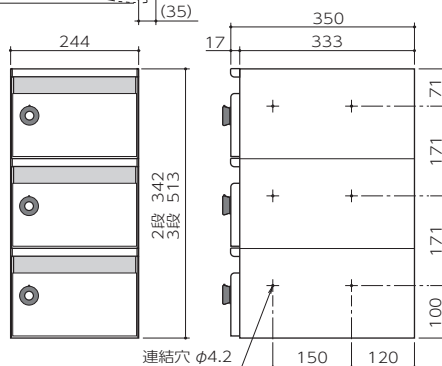
●施工図
