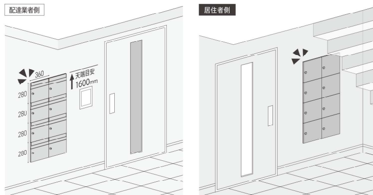
オートロックエントランス脳埋め込み設置イメージ (8世帯分)
