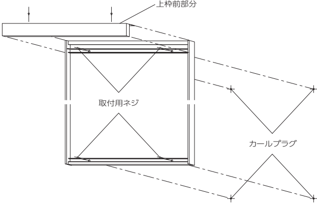
組立図
