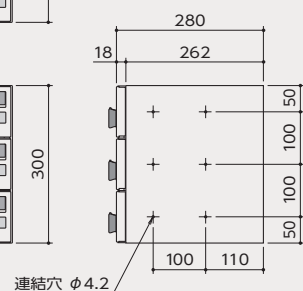
連結穴 \phi 4.2
