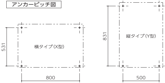
アンカーピッチ図
