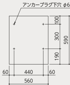
アンカーピッチ図
