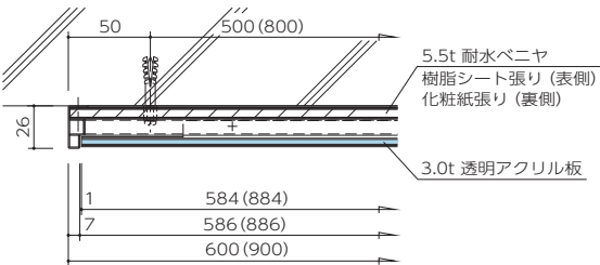
平断面
