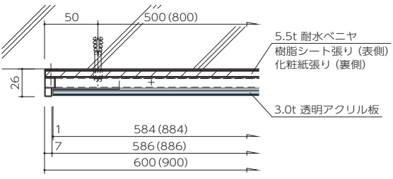
組立図
