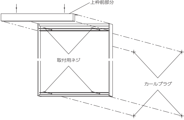
組立図
