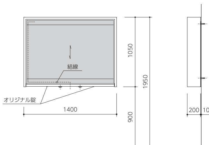
●PC4-W型
