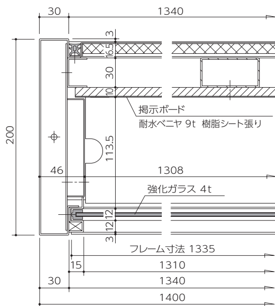
●平断面图
