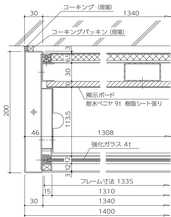
●平断面図
