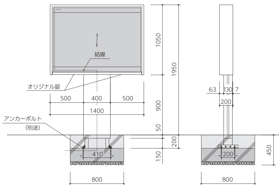
●PC4-P型
