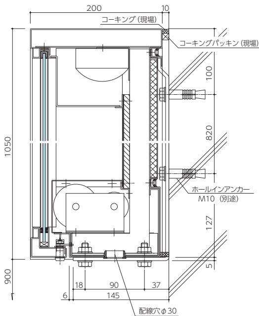
立断面
