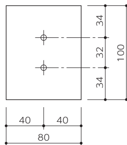
アンカーピッチ図
