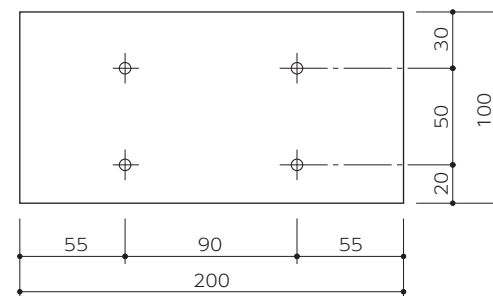
アンカーピッチ図
