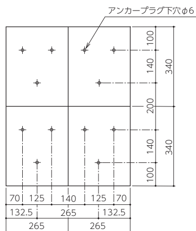
●アンカーピッチ図
