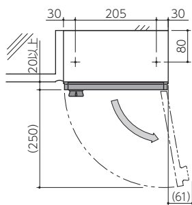
●施工図
