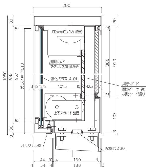
立断面
