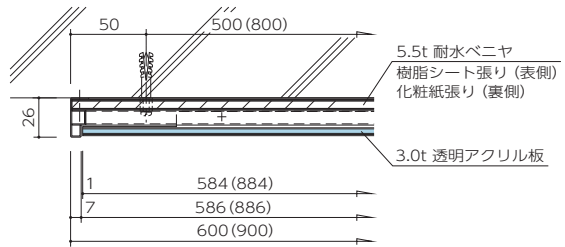
平断面
