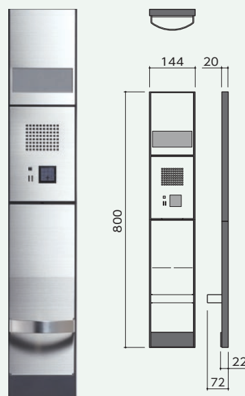
●スリムポーチT
