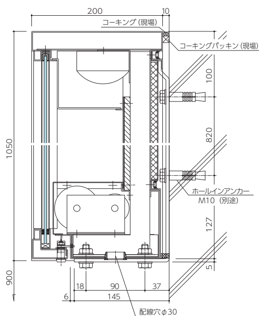
立断面
