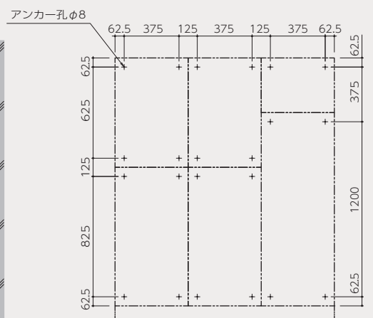
アンカーピッチ図
