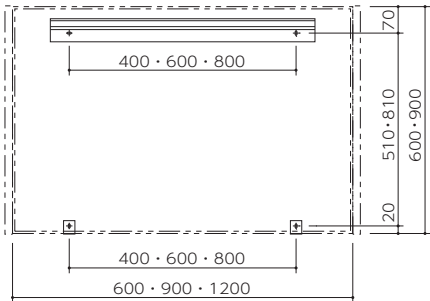
アンカーピッチ図
