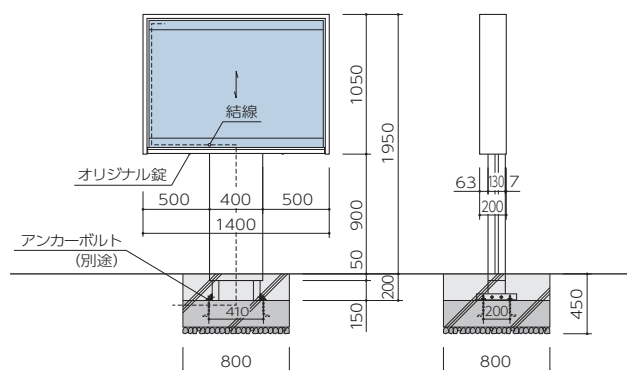
立断面
