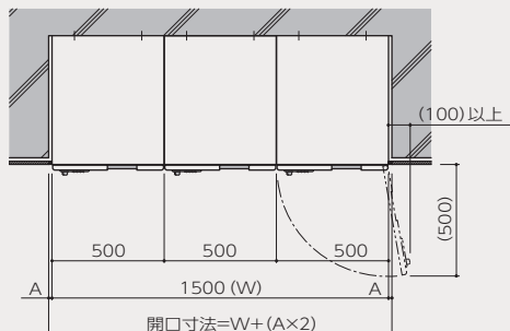
平面
