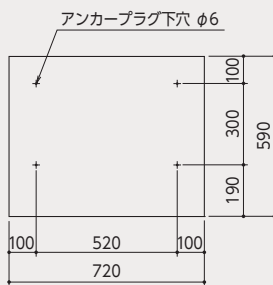
アンカーピッチ図
