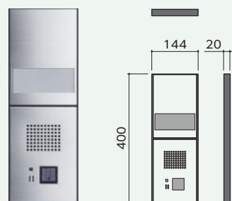
●スリムポーチS (室名札・インターホンパネル)
