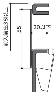
〔PS-1 装着断面〕
