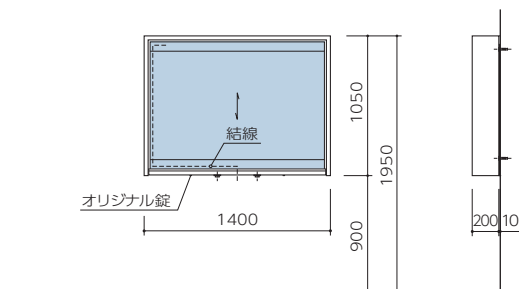
PC4-W / 壁付タイプ
