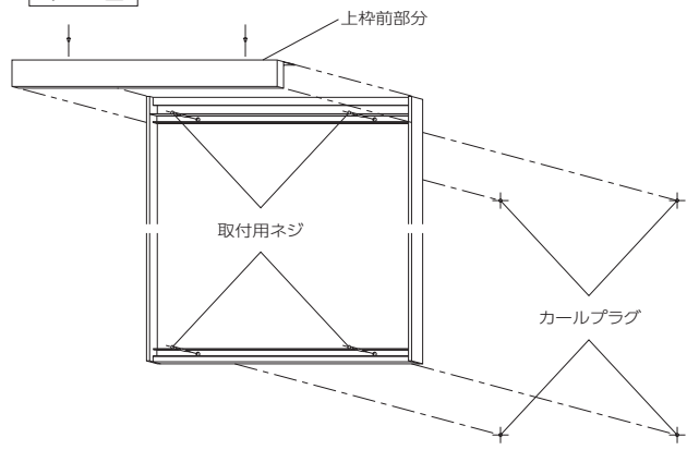
組立図
