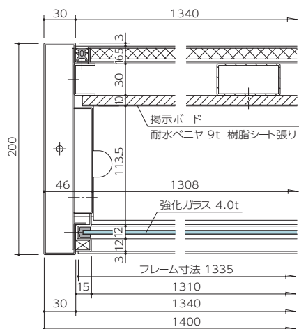
平断面
