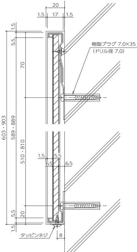
立断面
