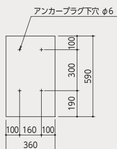
アンカーピッチ図
