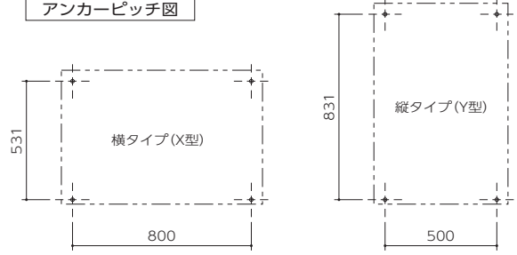
アンカーピッチ図
