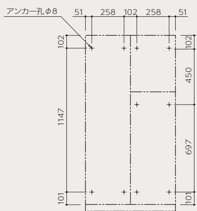
アンカーピッチ図
