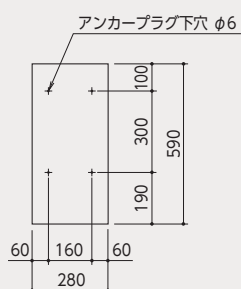
アンカーピッチ図
