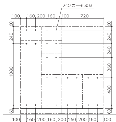
アンカーピッチ図
