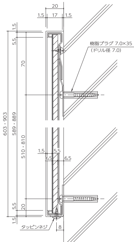
立断面
