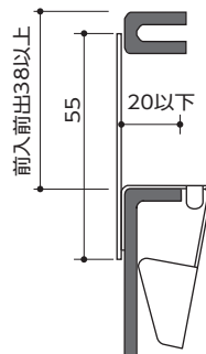
【PS-1 装着断面】
