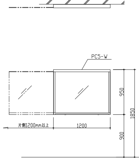
壁付タイプ
