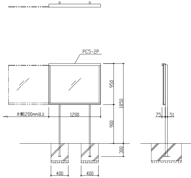
脚付タイプ
